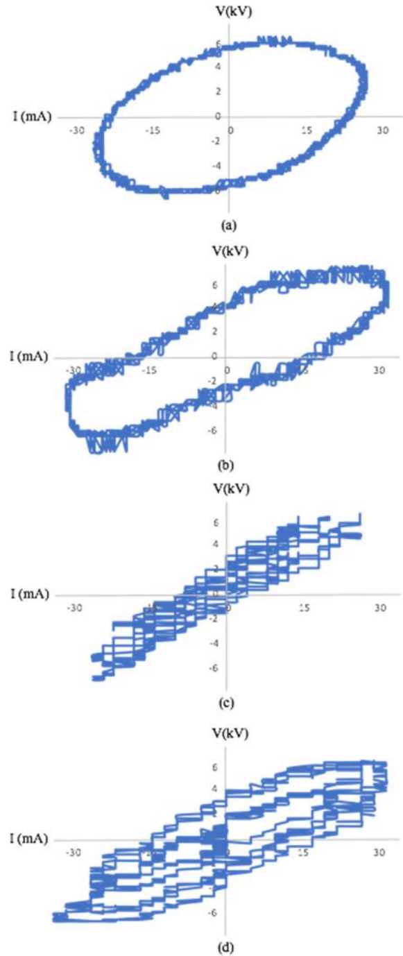
Fig. 6. Lissajous figures. (a) model I,(b) model II, (c) model III and (d) model IV
