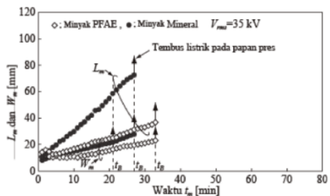
Gambar 4. L_m dan W_m sebagai fungsi waktu t_m pada berbagai level tegangan
