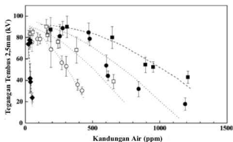
Gambar 2. Kurva tegangan tembus 2.5-mm dengan kandungan air pada minyak mineral (diamon hitam) dan berbagai turunan PFAE pada suhu kamar (~25 °C): C8-Me (persegi hitam), C12-Me (lingkaran hitam), C8-2EH (persegi putih), dan C12-2EH (lingkaran putih)
